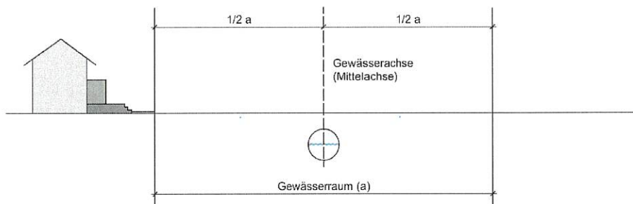
Messweise bei eingedolten Fließgewässern
