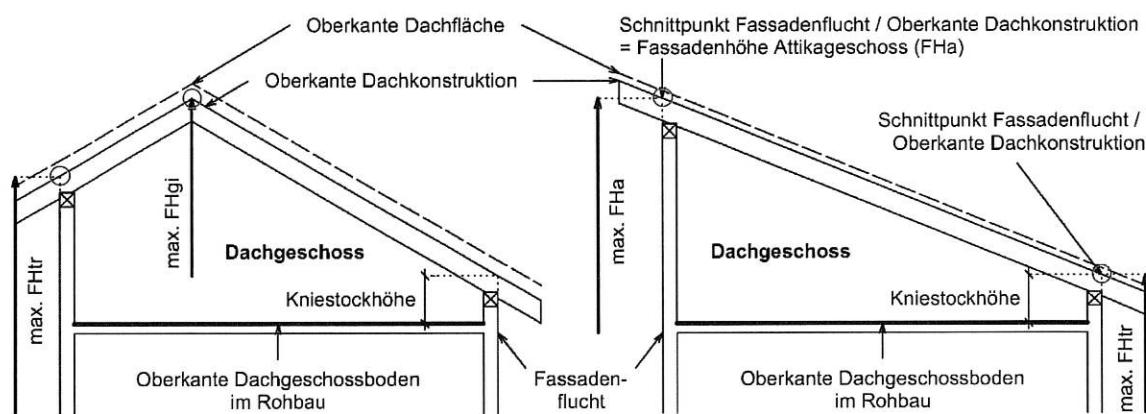
Grafik gemäss BMBV Figur 5.3 mit Anpassung; Die Fassadenhöhen (FHtr, FHgi, FHa) werden abgebildet.
