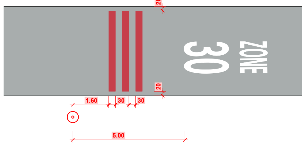
Detail Zoneneingang T30 1:100
